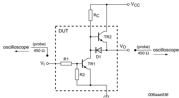
I_C = 0.05\text{ A}; I_B = 2.5\text{ mA}; R_C = 180\text{ }\Omega
